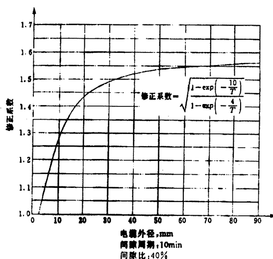
图3 间隙运行的修正系数
