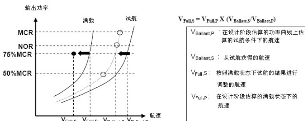
图 4.3.7.2 航速修正举例
