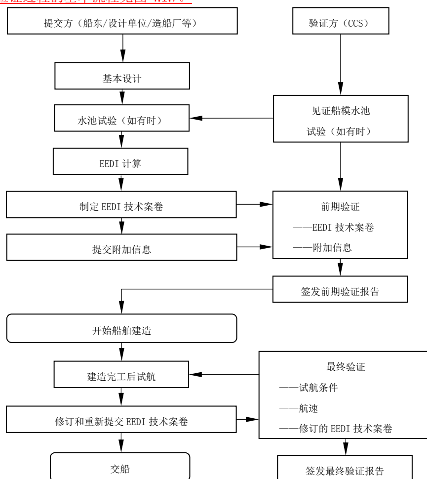
图 4.1.7 验证过程基本流程
