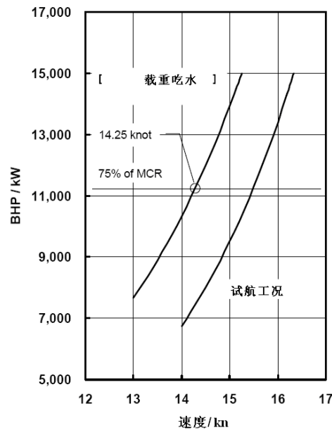
图3 功率曲线
