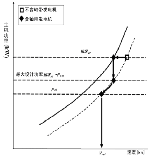
图 2.2.5 主机功率 P_{ME(i)} 的确定
