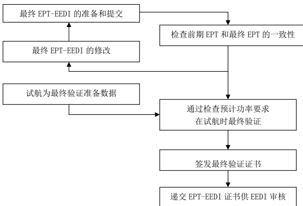
图 4.7.2 (2) EPT-EEDI 最终验证的基本流程
