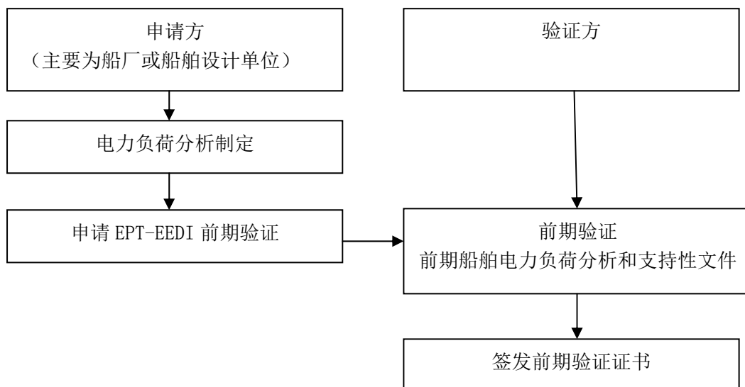
图 4.7.2 (1) EPT-EEDI 前期验证的基本流程
