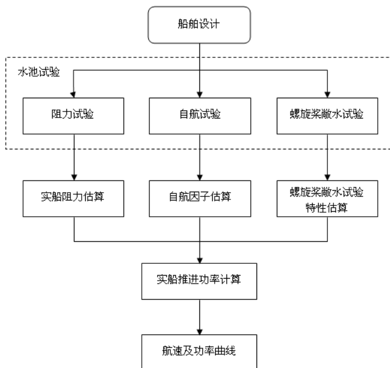
图 2 功率曲线估算过程流程图
